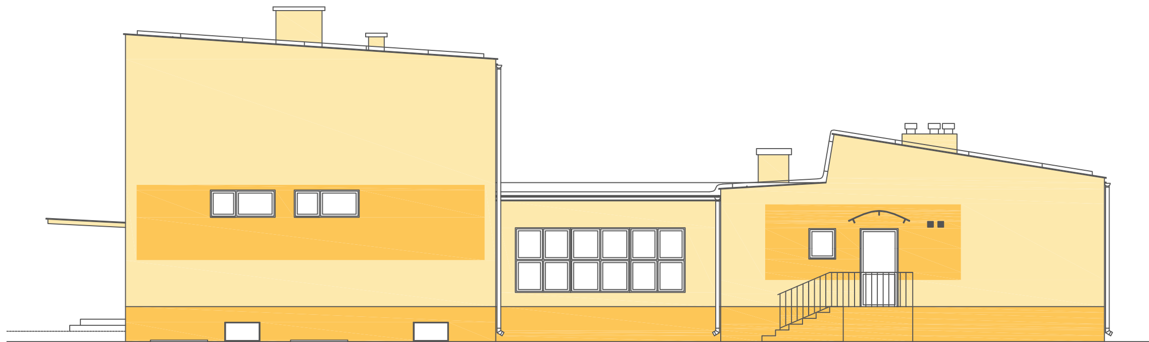
ELEWACJA POŁUDNIOWA - 4
